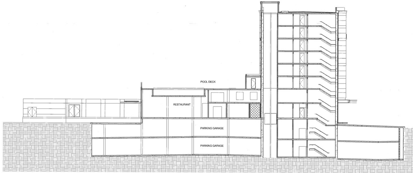
3 Longitudinal Section 'B' 3/32" = 1'-0"
